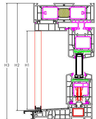
Przekrój (widok z boku)
