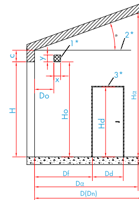
Przekrój boczny
